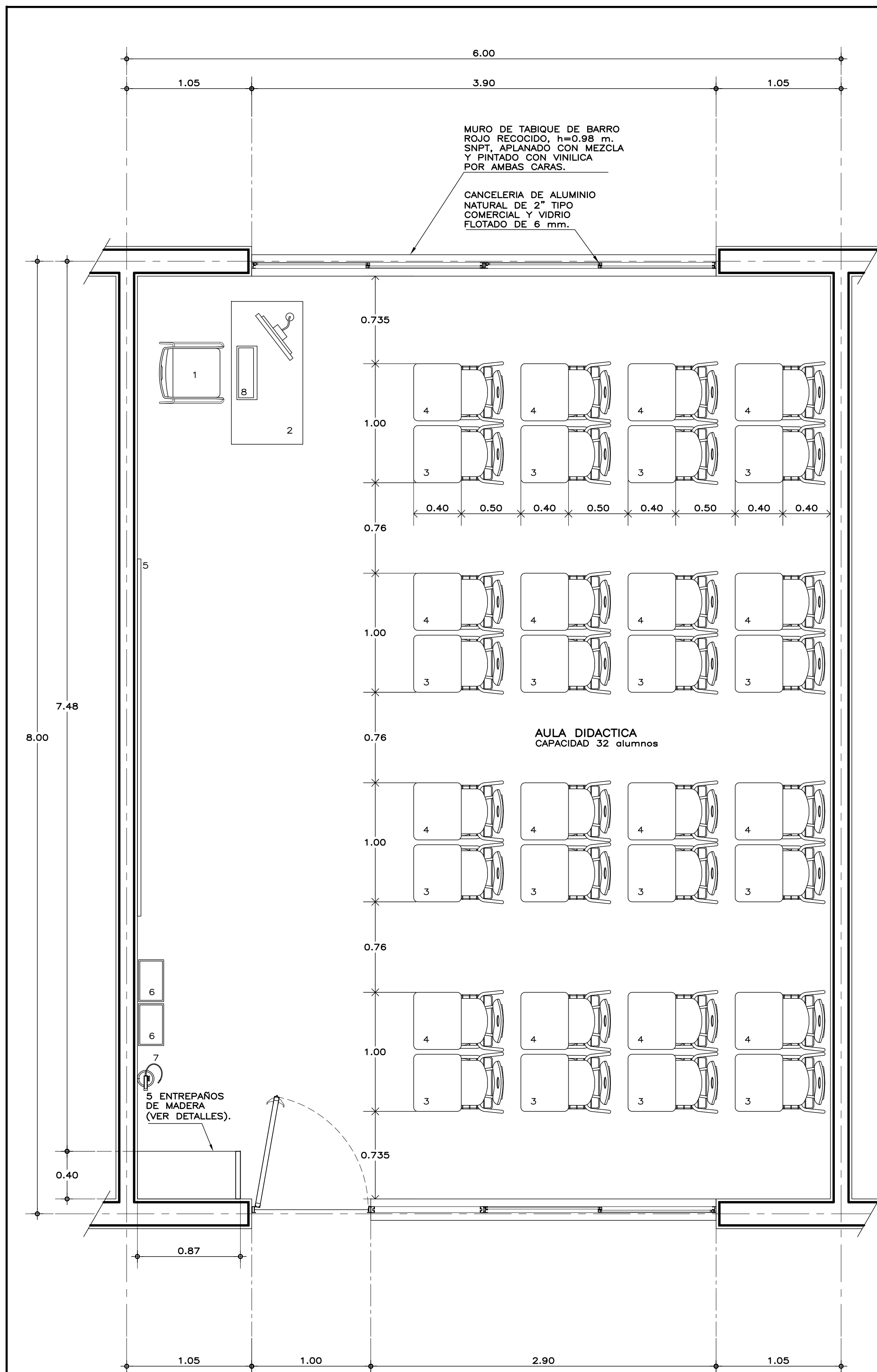
PLANTA ARQUITECTONICA OPCIONES DE AMUEBLADO 1 Y 2
