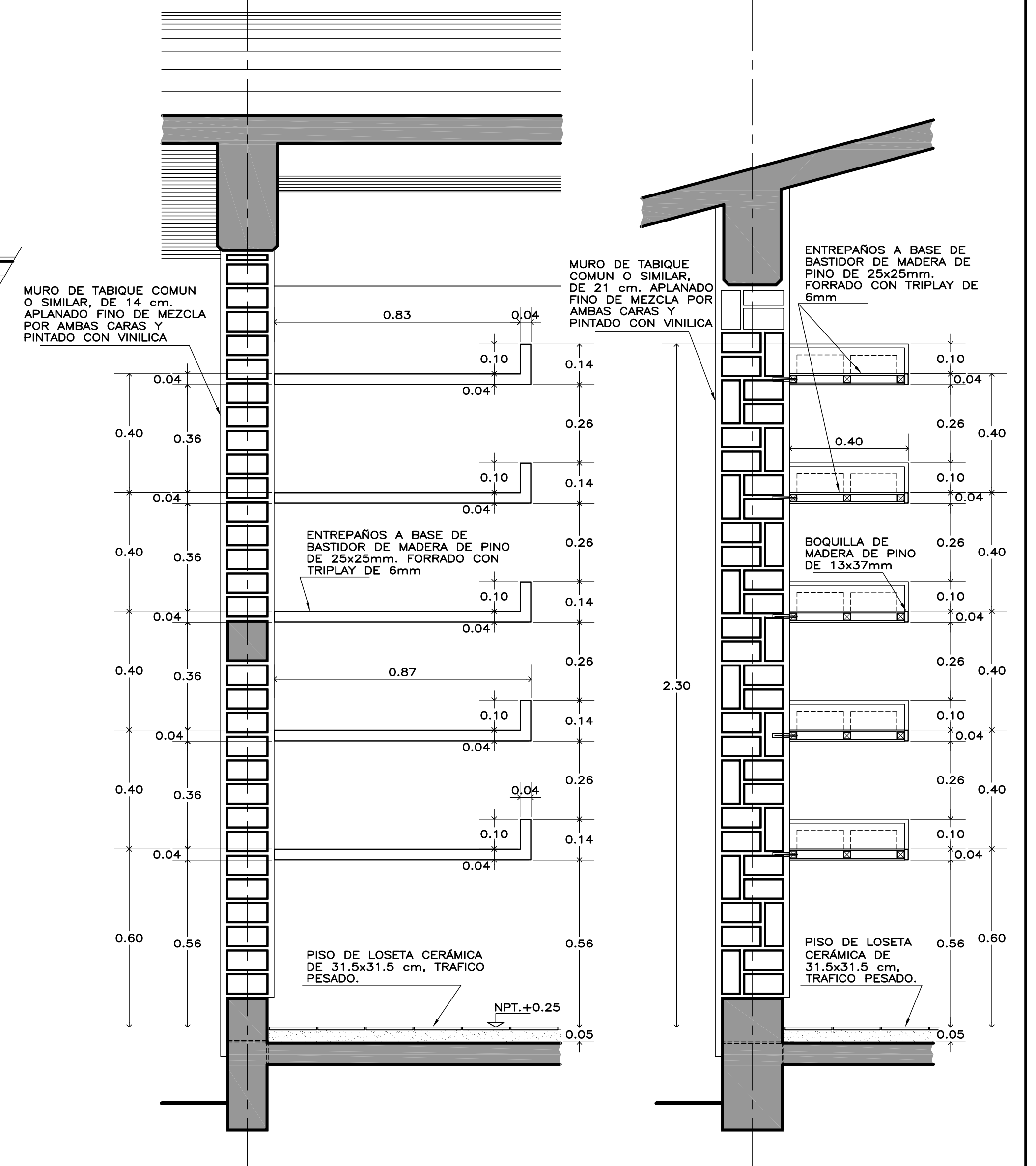
ALZADO ENTREPAÑO S/ESC.
