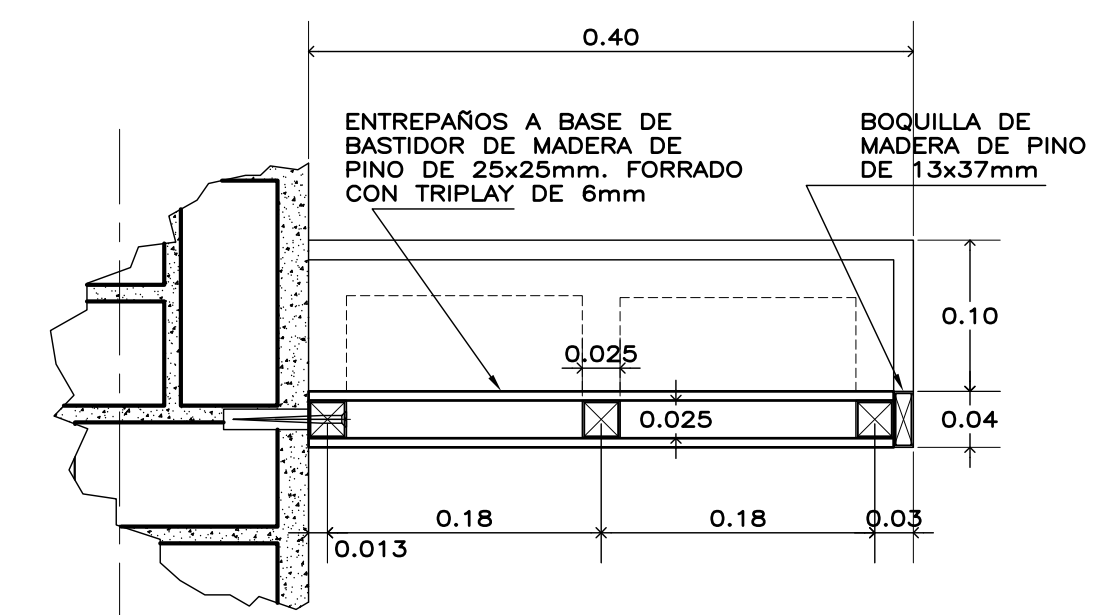
DETALLE ENTREPAÑO e s c. 1 : 1 0
